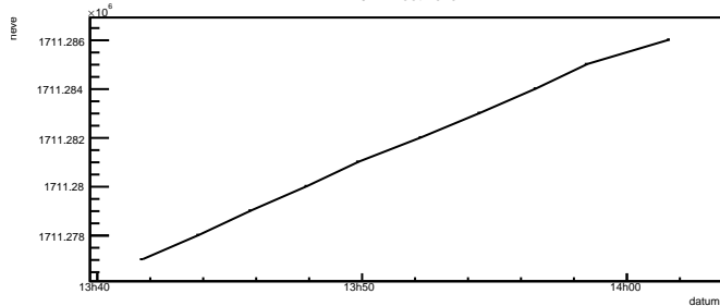
r0127.root neve
