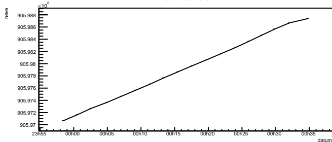
r0074.root neve
