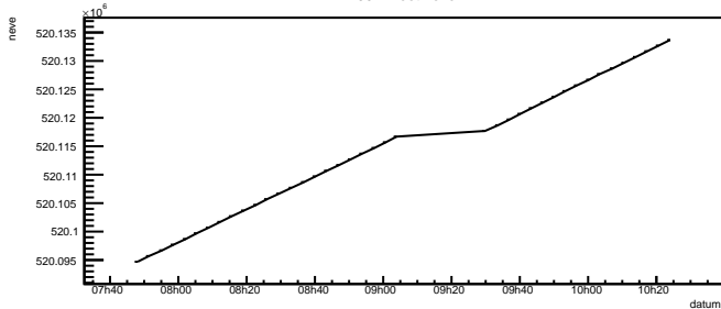
r0047.root neve
