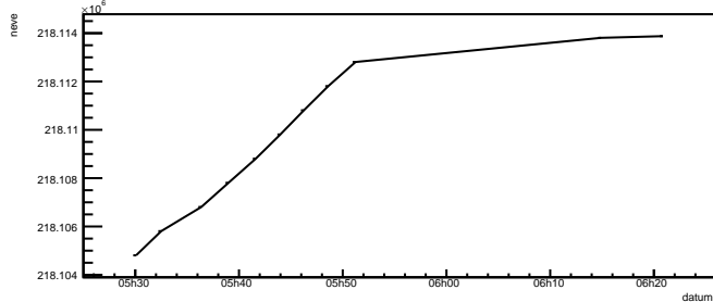
r0026.root neve
