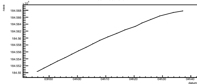
r0024.root neve
